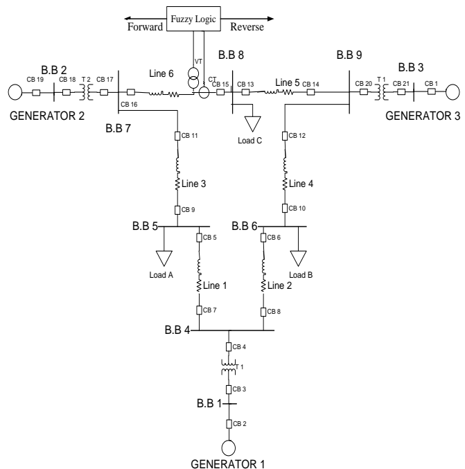
Fig. 1. IEEE 9-Bus Grid
